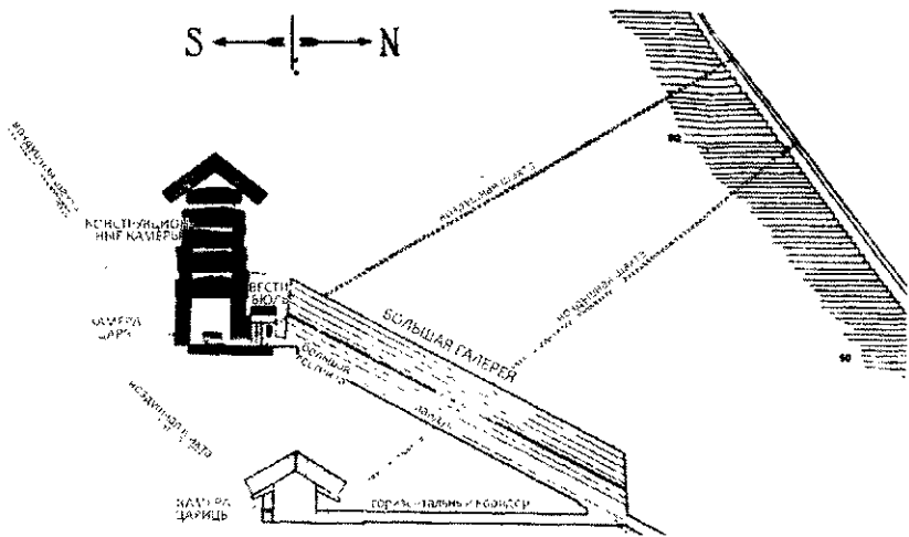
Поперечный разрез с указанием воздушных шахт
