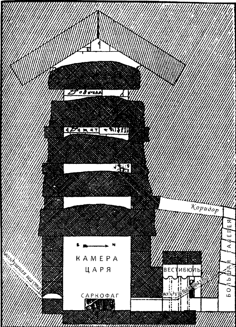
ВЕРТИКАЛЬНЫЙ РАЗРЕЗ КАМЕРЫ ЦАРЯ (вид на запад), вестибюля и конструктивных камер Говарда Визе с указанием формы блоков (прямые линии обозначают известняк, перекрещивающиеся линии обозначают гранит)
